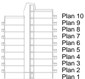
PRINCIPSEKTIONER
